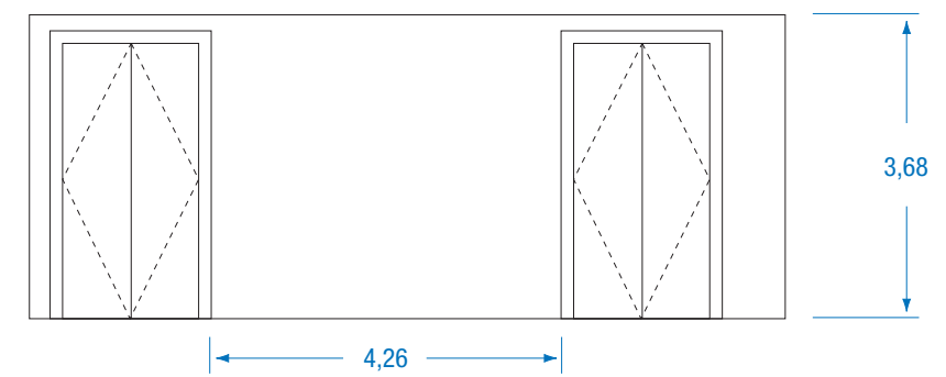
Alzado lateral dereito
